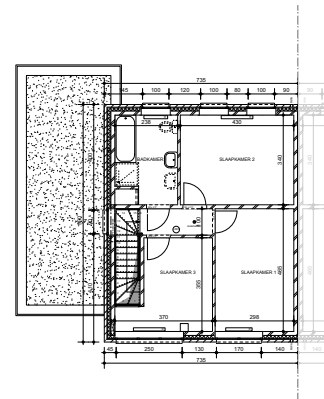
EERSTE VERDIEPING_schaal 1.100
